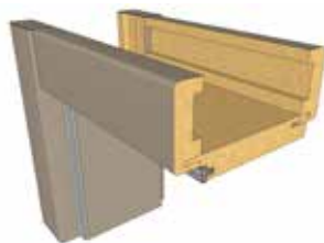
Řez obložkovou zárubní pro otočné dveře - na TUPO síla zdi od 5 cm, límce 6 cm
